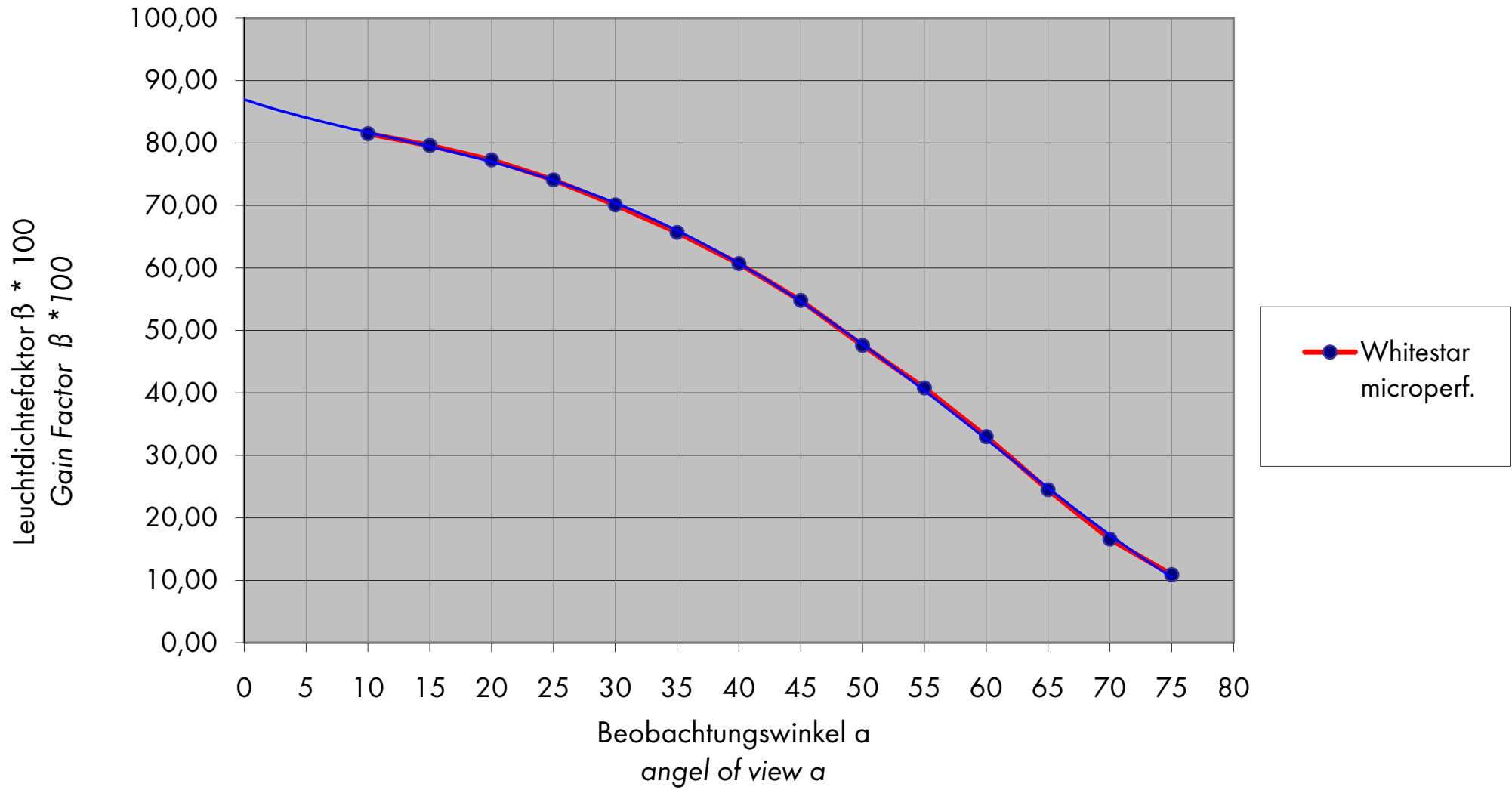
Projektionsfolie WHITESTAR MICROPERF - Reflexion nach DIN 19045-4 projeccion screen WHITESTAR MICROPERF - reflexion acc. to DIN 19045-4
