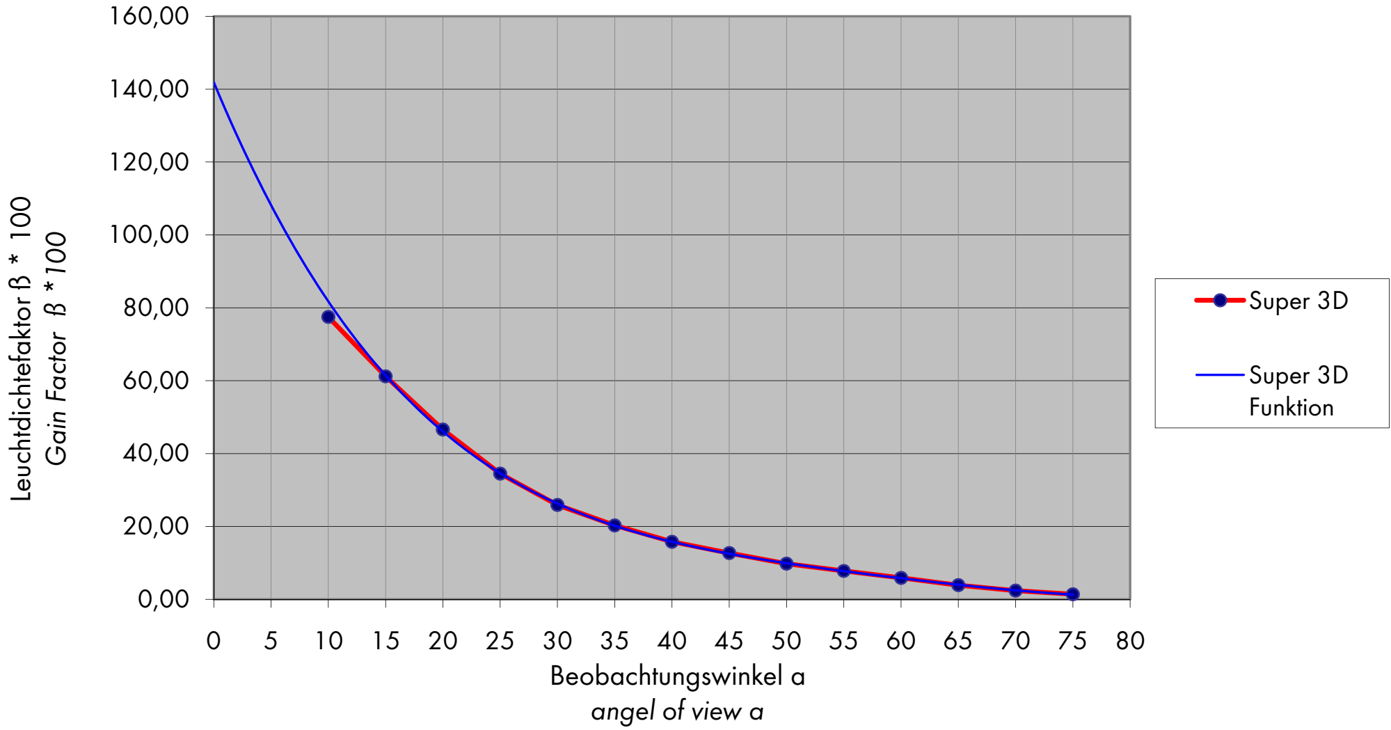
Projektionsfolie SUPER 3D (3D-Seite)- Reflexion nach DIN 19045-4 projection screen SUPER 3D (3D-Seite) - reflexion acc. to DIN 19045-4
