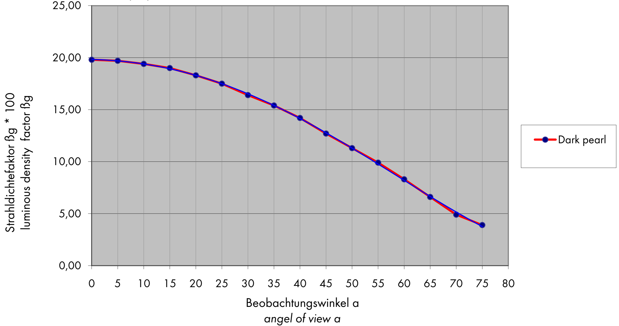
Projektionsfolie DARK PEARL - Transmission nach DIN 5036-3 projecion screen DARK PEARL - transmission acc. to DIN 5036-3
